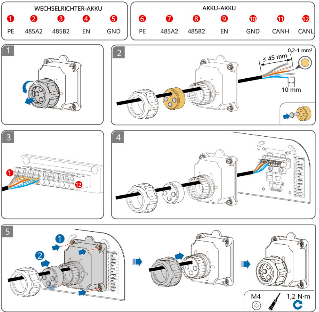
Abbildung 5-6 Signalanschlussverbindungen
